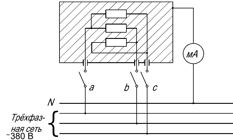
Рисунок 4 — Схема измерения тока утечки
