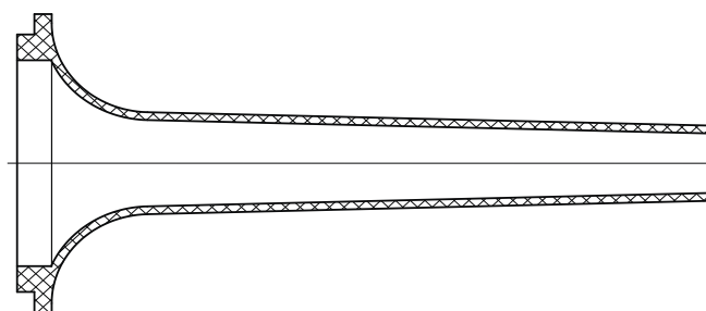
Рисунок 7 – Насадка
