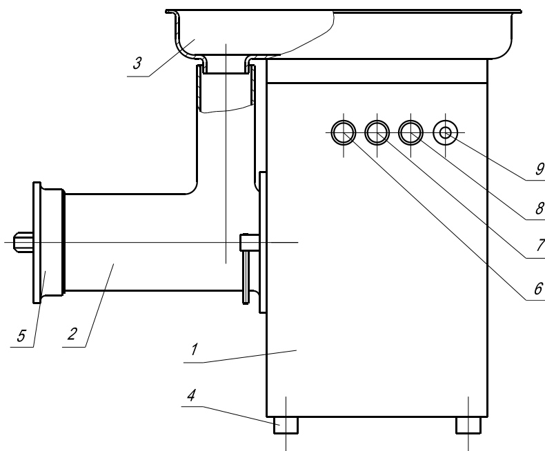
1 - кожух; 2 - мясорубка в сборе; 3 - чаша в сборе; 4 - основание (на опорах); 5 - гайка; 6 - Кнопка «Пуск»; 7 - Кнопка «Стоп»; 8 - Кнопка «Ревёрс»; 9 - Лампочка «Сеть»
