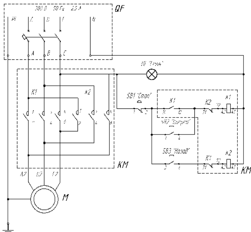
QF - Выключатель автоматический; KM - Пускатель магнитный; M - Электродвигатель; SB1 - Кнопка «Стоп»; SB2 - Кнопка «Пуск»; SB3 - Кнопка «Реверс»; HL - Сигнальная лампочка
