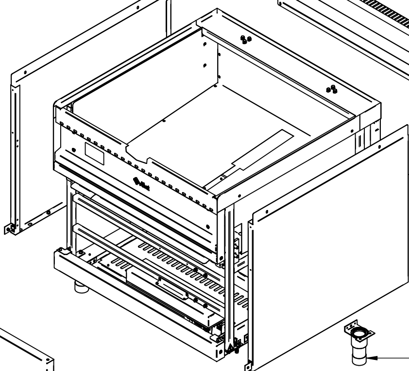
Стенка боковая (левая) 60001009789
