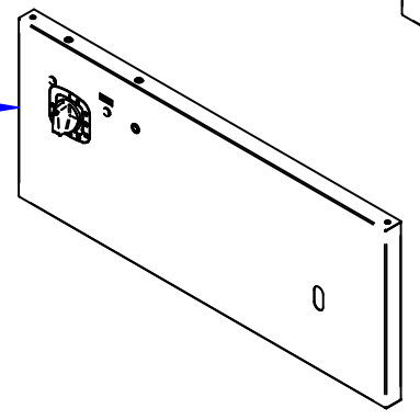
Панель передняя ЭСК-90-0,47-70-4.003 РС 00001002725
