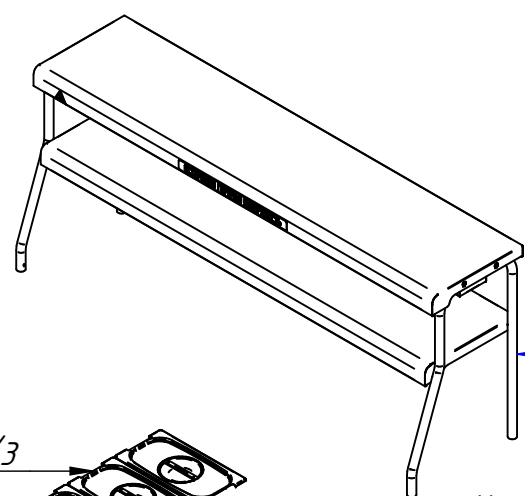
Полка двойная (подогреваемая) (в сборе) 1500 мм ЭМК-70КМ-01.2501.001 РС 21001008362
