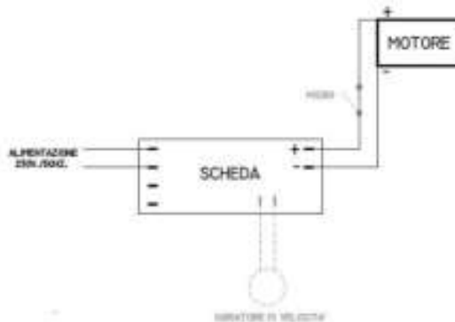
Рис. № 5 - Однофазная электрическая схема
