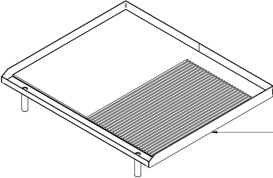
Плита жарочная (в сборе) AKO-90.05.01.000СБ 21000001493
