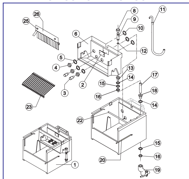
CIRCUITO IDRAULICO
