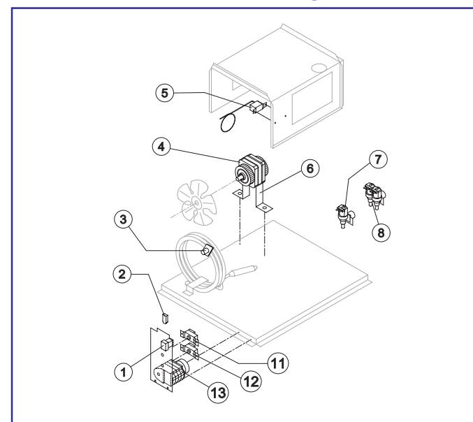
PARTI ELETTRICHE
