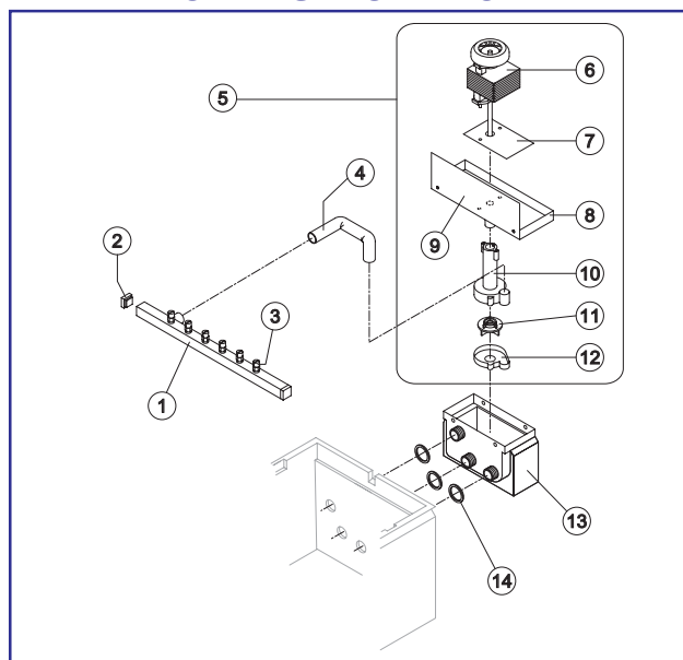
POMPA SPRUZZATORE
