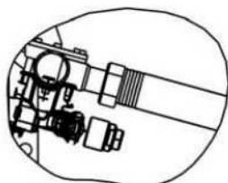
CONEXION ENCIMERA-HORNO MEDIANTE TUERCA Y JUNTA 1/2" DETALLE A ESCALA 1/4
