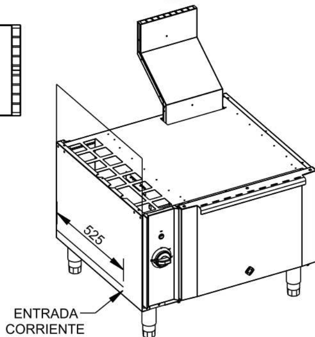
DETALLE A
