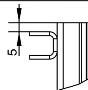
DETALLE A ESCALA 1/2
