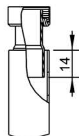
MUY IMPORTANTE SOLDADURA CON PLATA DETALLE B ESCALA 1/2
