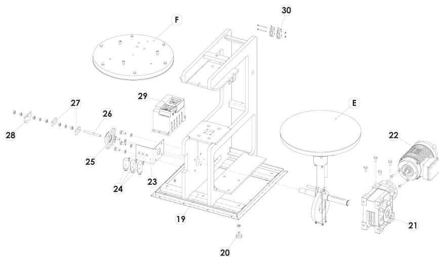
Det. C
