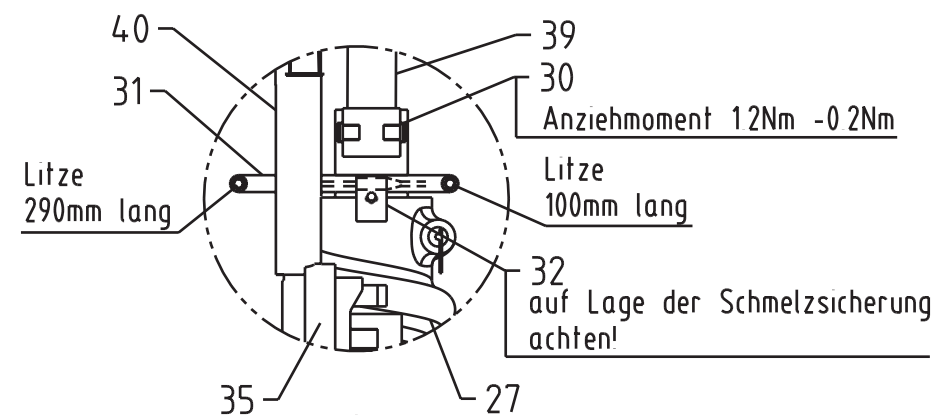
Montage Schmelzsicherung/Temperaturregler
