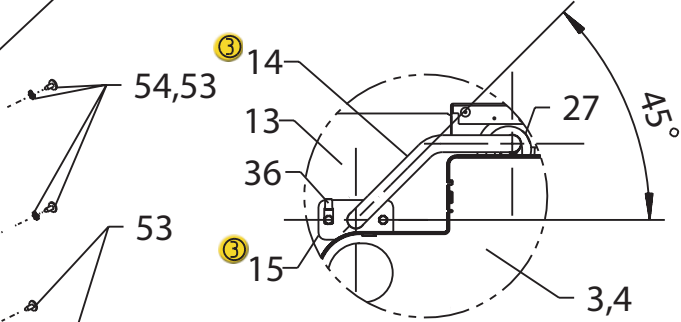
Montage Ueberlauf
