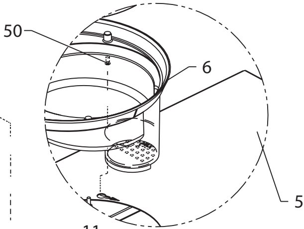
Montage Ueberlauf
