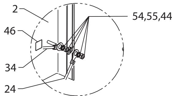
X Erdungsaufbau
