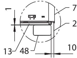
Positionierung Typenschild
