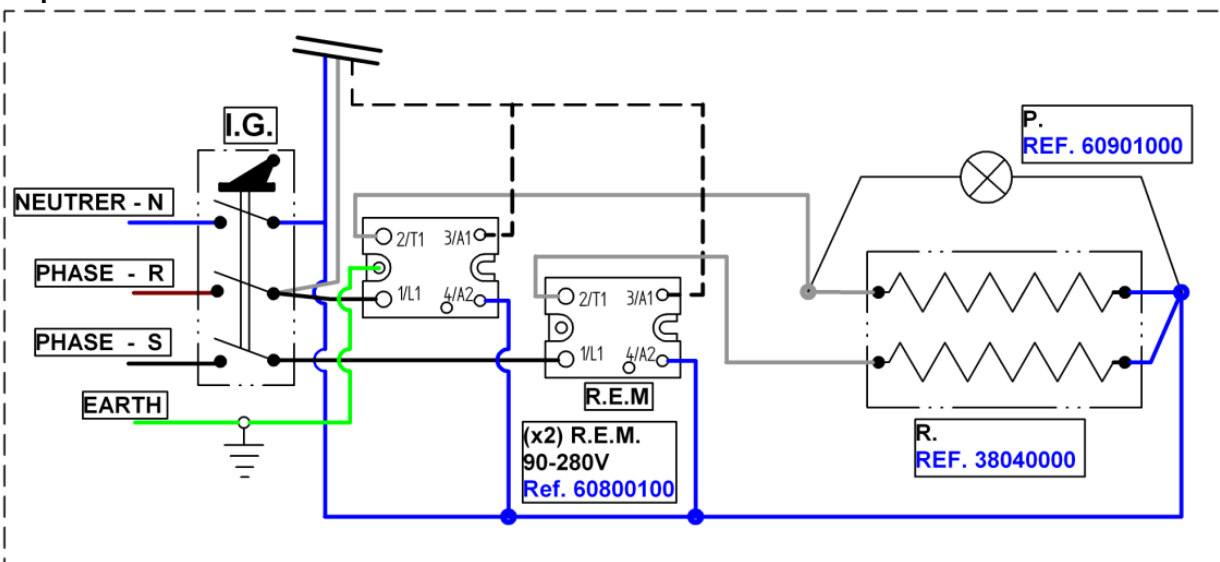
Esquema eléctrico 3GR 380V 2F+N.
