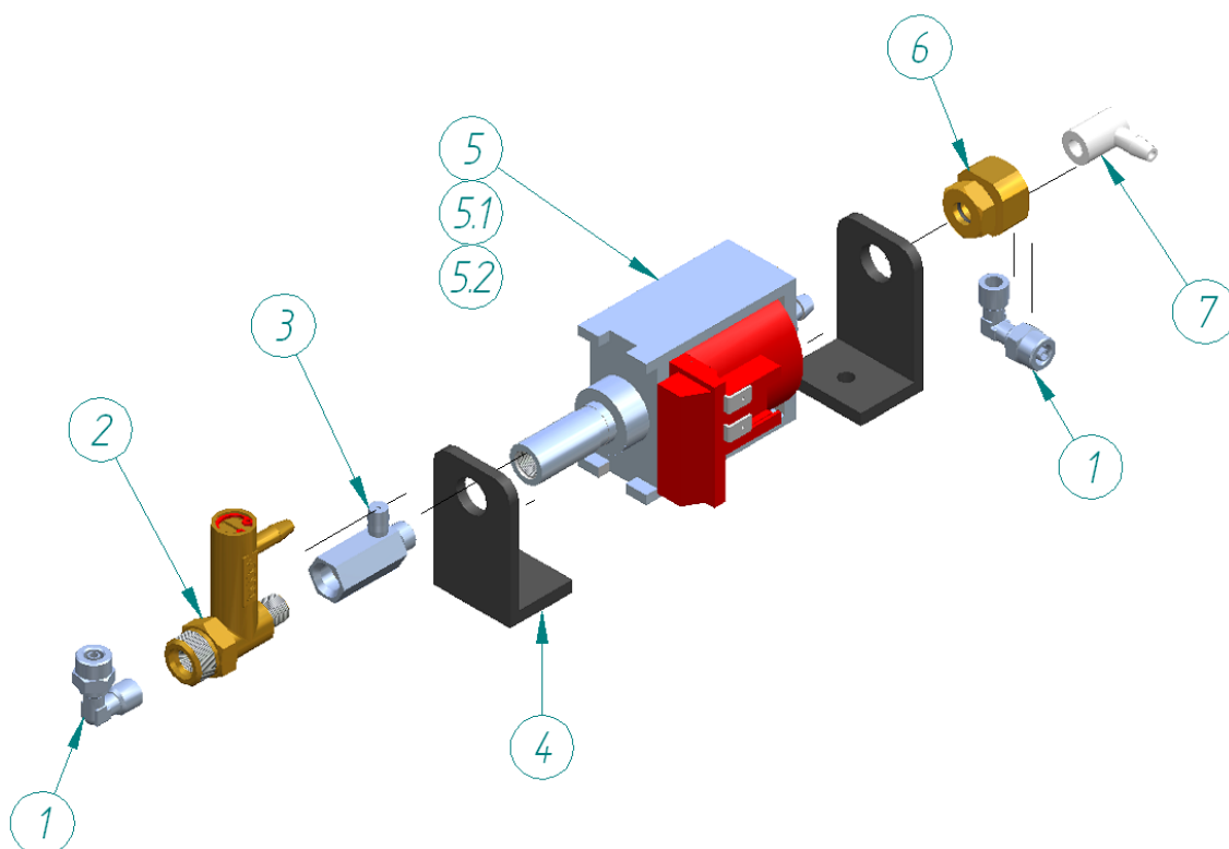
CONEXIÓN DEPÓSITO.
