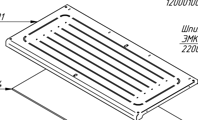
Плита СХС(М)-70.24.17.00.00.003 50000002815
