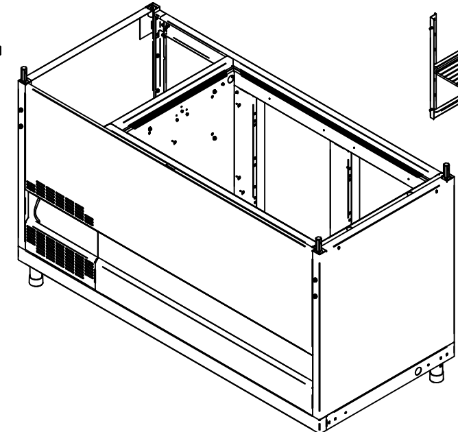
Направляющая линии "Аста" 1500 мм в сборе ЭМК70К-50-01СБ 21000002893
