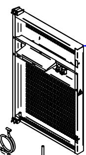
Панель управления ПВВ(Н)-70КМ-С-01-ОК.4962.002 РС 60001012996
