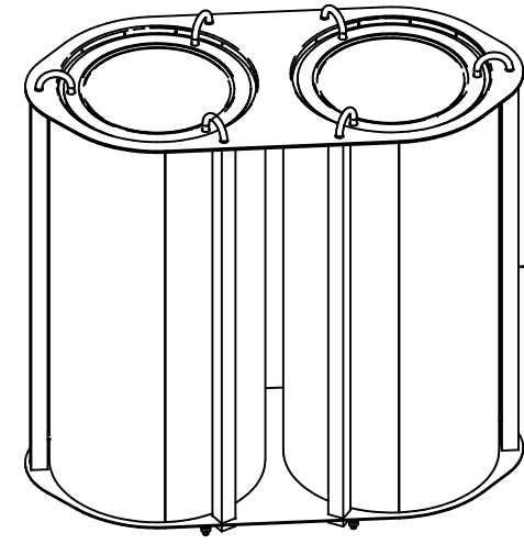
Кассетница (в сборе) ПТЭ70КМ-80.7546.37.00.000СБ 21001003625
