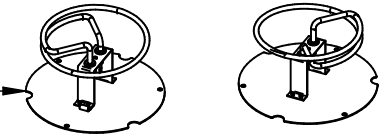
Блок нагревательный (2 шт.) ПТЭ70К-80.02.000СБ 21001012894
