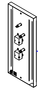
Панель управления ПТЭ-70Т-80.5761.001 РС 21001002898
